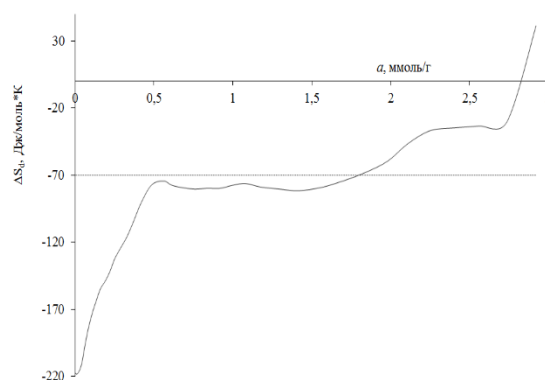
2-Расм. 303 К да гибрид диацетатцеллюлоза-кремнезем бионанокомпозицион материалга сувни адсорбциясининг энтропияси: горизонтал штрихланган чизик - ўртача моляр интеграл энтропия. Суюқ сувнинг энтропияси нолга тенг.
