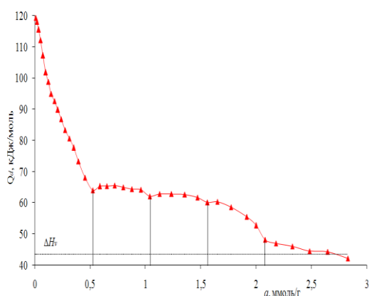
1-Расм. 303 К да гибрид диацетатцеллюлоза-кремнезем бионанокомпозицион материалга сувни адсорбциясининг дифференциал иссиқликлари: горизонтал штрихланган чизик - сувни конденсация иссиқлиги.
