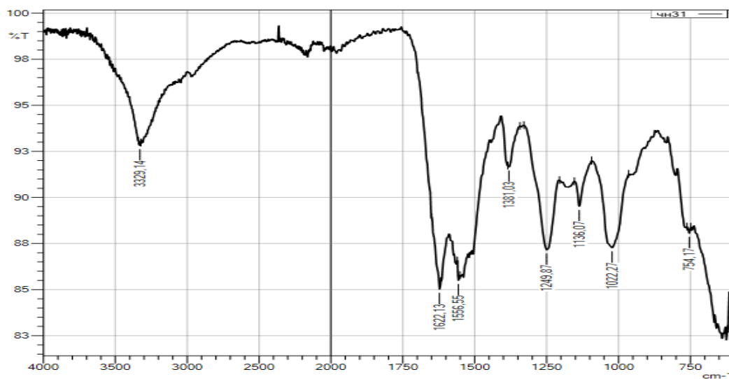
1-Rasm. karbamid formaldegid va ditizon bilan modifikatsiyalangan olingan sorbentning IQ-spektrlari
