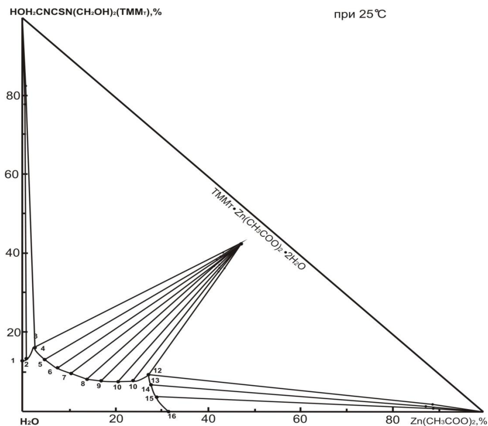
1-расм. 25^\circ\text{C} да Триметилолтиомочевина – рух ацетат – сув тизимининг эрувчанлик диаграммаси
