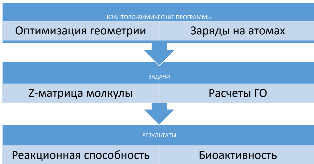
Рис 1. Возможности квантово-химических программ
