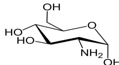
Glyukozamin sulfatning kimyoviy tuzilishi
