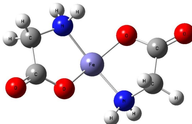
Рисунок 1. Строение молекулы бисглицината железа на программе
