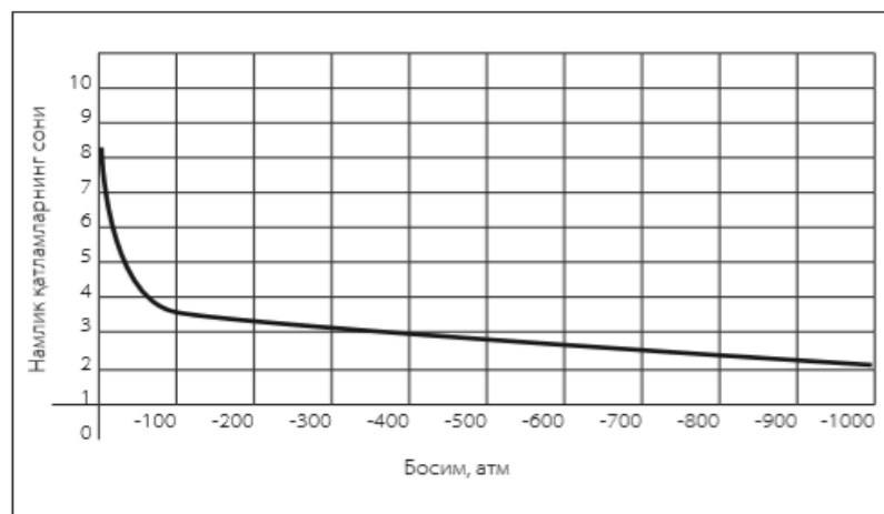
1.1-rasm Tuproq substrati zarrachalari qatlamlaridan har xil uzoqlikda joylashgan qatlamlardagi suv bosimi.
