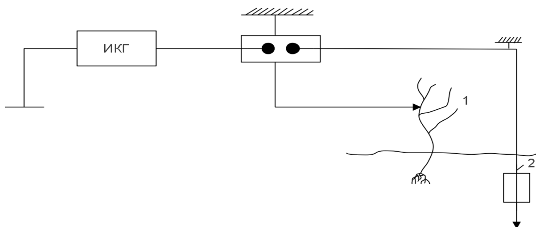
2-rasm. O'simlik hisobiga yashayotgan zararli begona o'tni quritish sxemasi 1-o'simlik; 2-elektrod. ИПК- импульс кучланish generatori.
