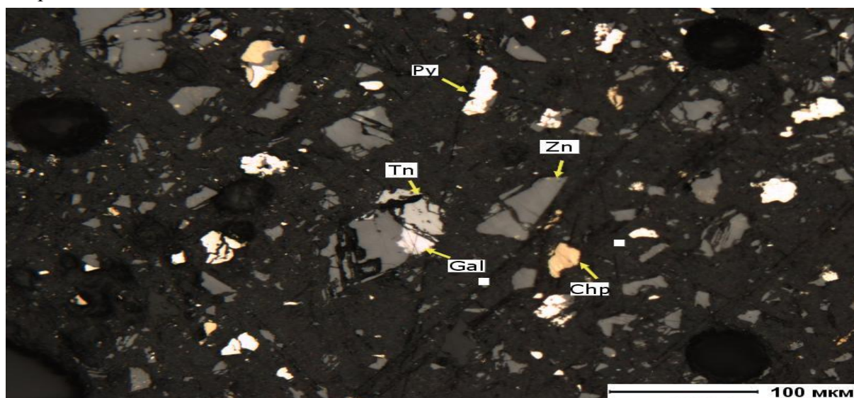
Рис.1. Минералогический анализ цинкового концентрата месторождения Кемперсай
