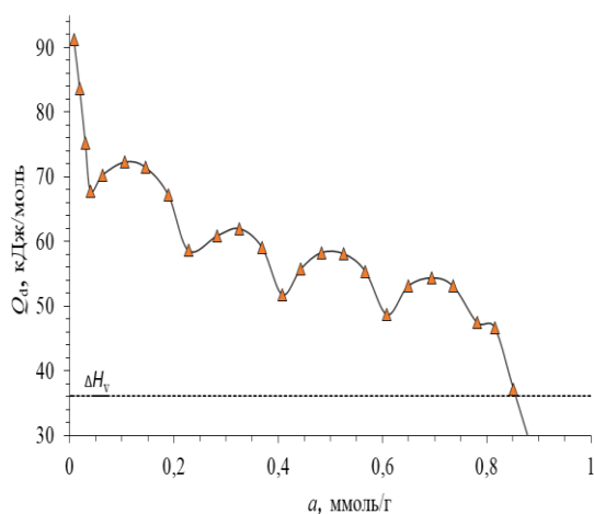
3-расм. 303 К да гибрид диацетат-целлюлоза-кремнезем бионанокомпозицион материалга бензолни адсорбциясининг дифференциал иссиқликлари: горизонтал штрих чизик – бензолни конденсация иссиқлиги.
