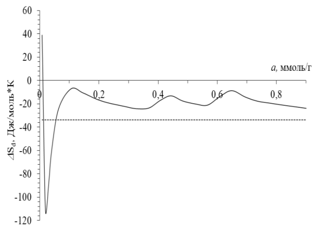
4-расм. 303 К да гибрид диацетатцеллюлоза-кремнезем бионанокомпозицион материалга бензолни адсорбциясининг энтропияси: горизонтал штрих чизик – ўртача моляр интеграл энтропия; суюқ бензолнинг энтропияси нолга тенг деб қабул қилинган.
