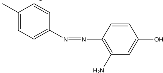
1-rasm. 6-metilpiridel-2-azo-m-aminofenol molekulası.
