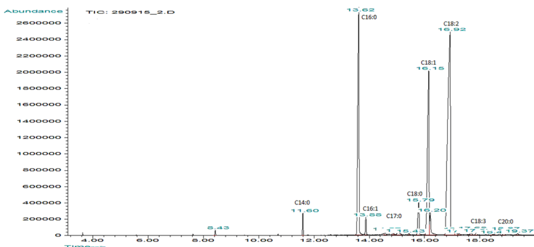
Рasm.2. ГХ – Амарант мойидаги ёғ кислоталар хроматограммаси
