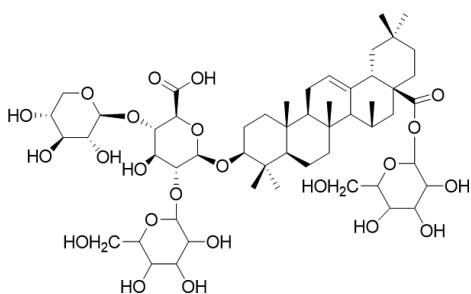
Рис. 1. Структурные формулы Салсолосидов С, Д и Е.
