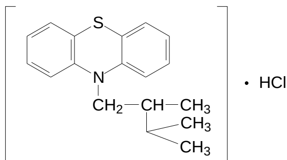
Схема 1. Химическое строение Трифтазина (Triftazin)
