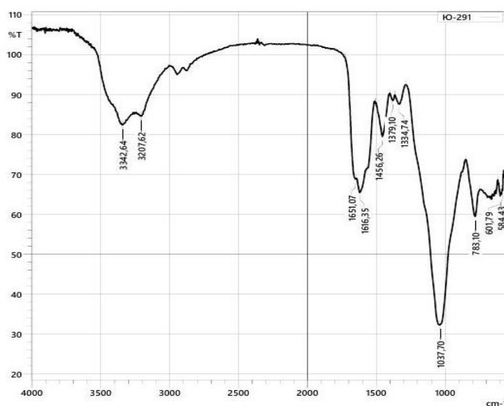
2-Rasm. SGEC-30 namunasining IQ-spektri
