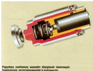
В) Pompacz pistoletowy Гидропорка
